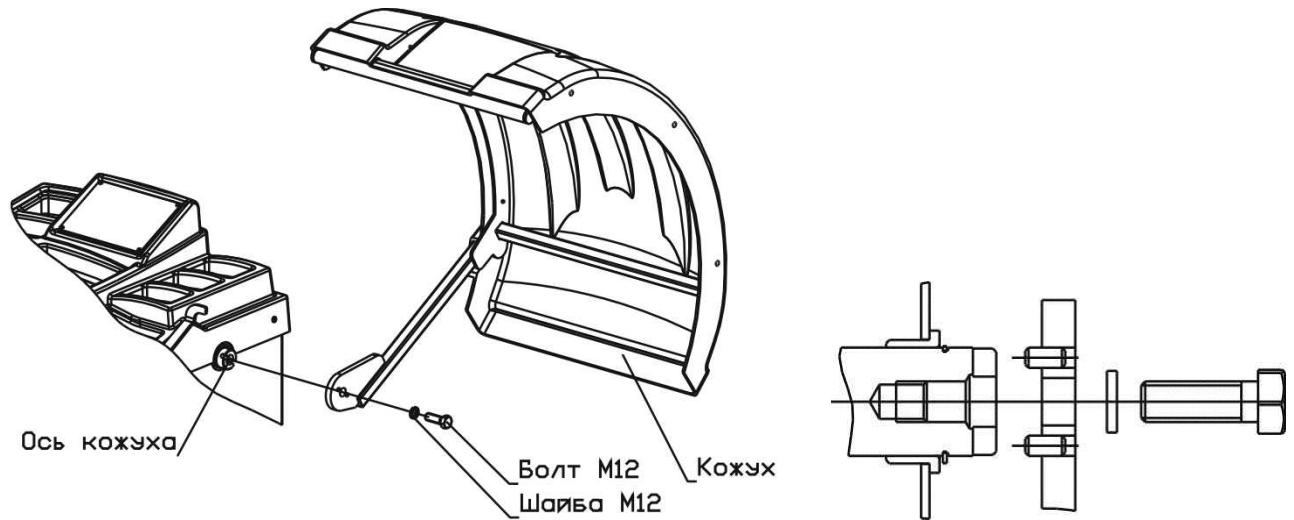
Рисунок 4.7 – Монтаж кожуха
